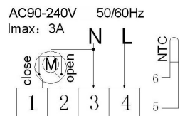
Vízfűtés kapcsolási rajza (ne csatlakoztassa a motoros szelep "close 4" terminálját)
