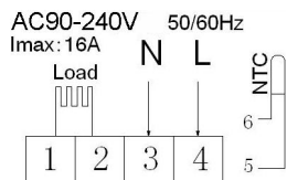
Elektromos fűtés kapcsolási rajza
